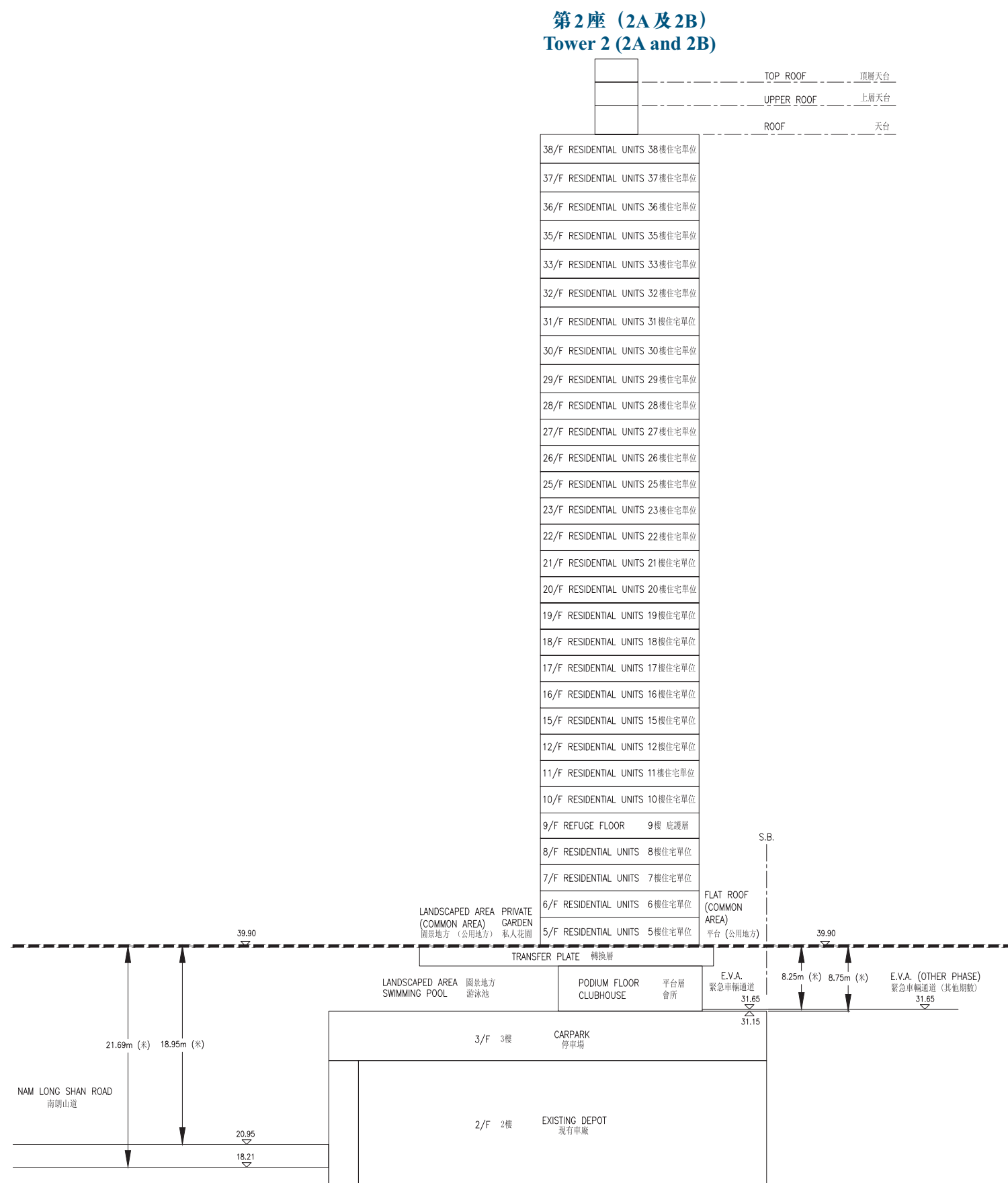
橫截面圖 B Cross-section plan B
